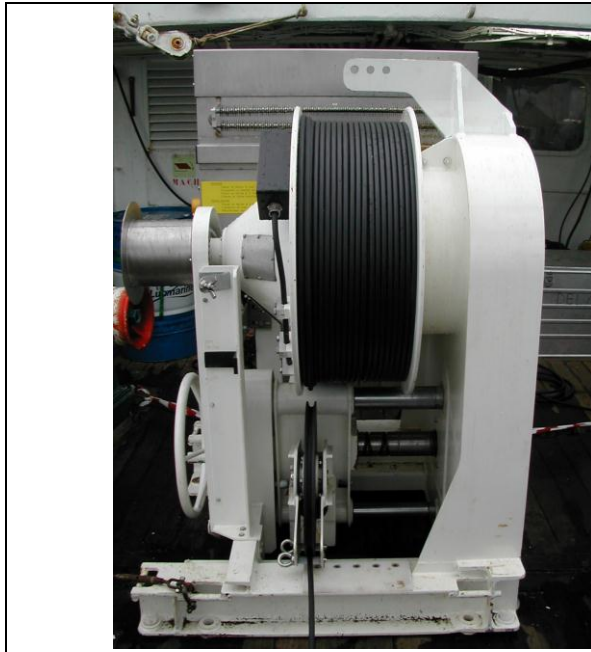
Treuil électro-opto-porteur à bord du Gwen Drez
