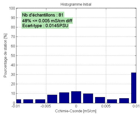
Figure 7 : Histogramme des écarts en conductivité avant ajustement.
