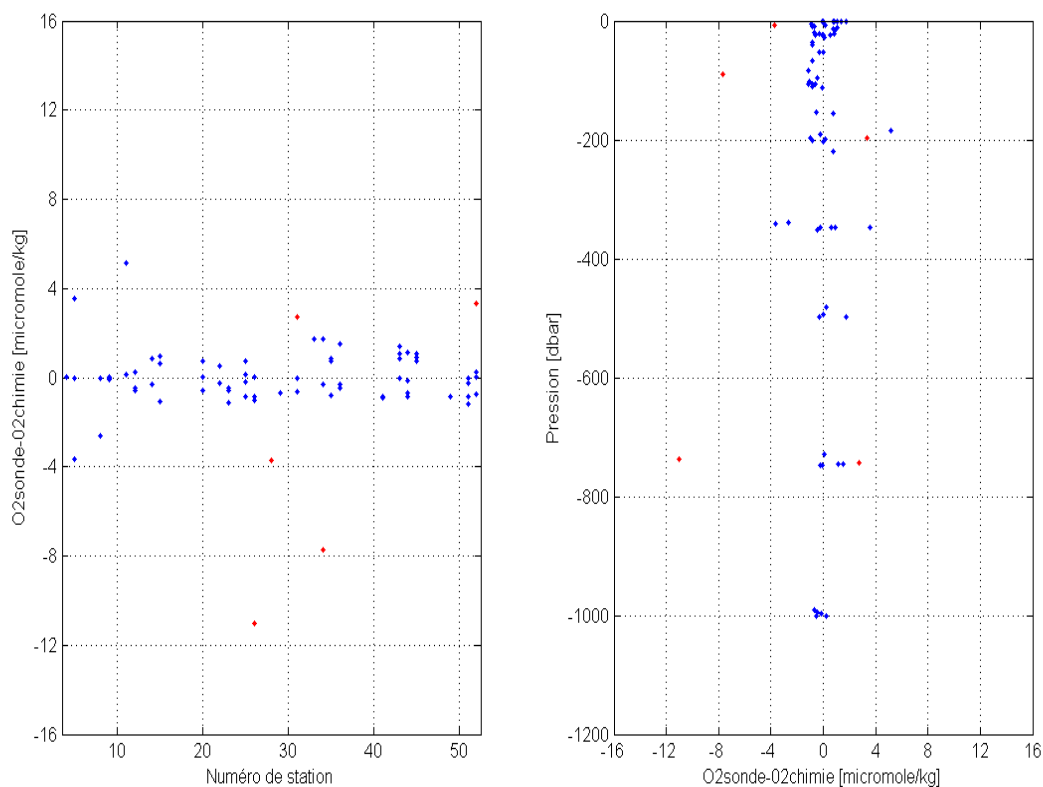
Figure 13 : Ecart en oxygène dissous (chimie-sonde) sur l'ensemble des stations après ajustement.
