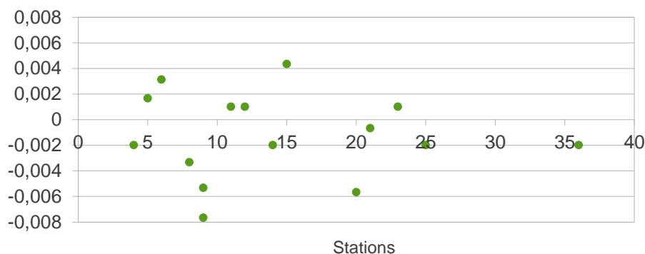
Figure 3: Ecart de salinité entre deux bouteilles fermées au même niveau en fonction du numéro de station à laquelle a été réalisé le doublet
