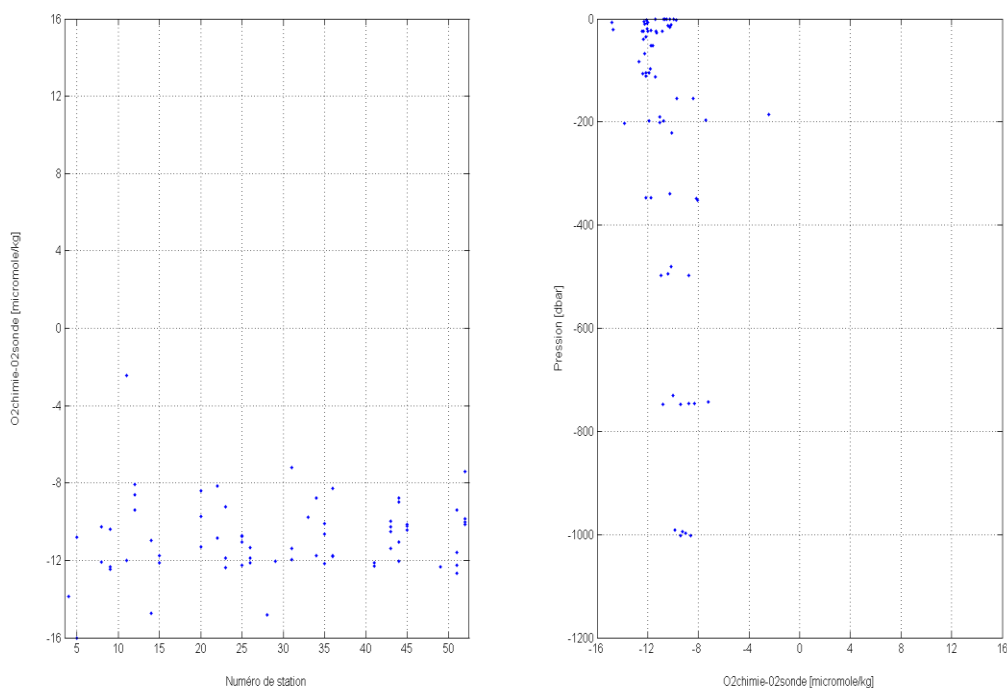
Figure 12 : Ecart en oxygène dissous (chimie-sonde) sur l'ensemble des stations avant ajustement.
