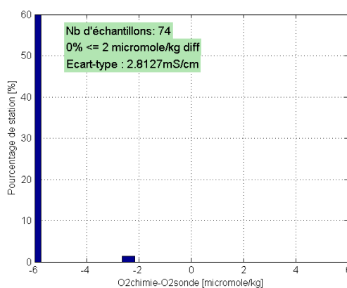
Figure 11 : Histogramme des écarts en oxygène dissous avant ajustement.
