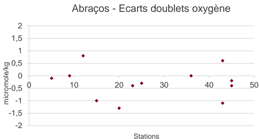
Figure 5: Ecart en oxygène dissous entre deux bouteilles fermées au même niveau en fonction du numéro de station à laquelle a été réalisé le doublet
