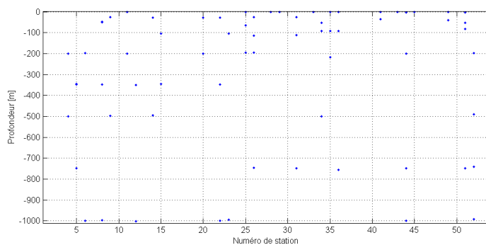
Figure 1 : Répartition des prélèvements pour analyse de l'oxygène dissous effectués au cours de la campagne ABRAÇOS.
