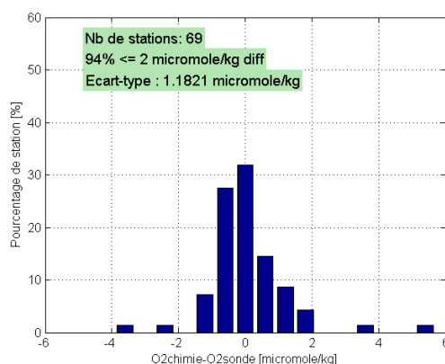
Figure 14 : Histogramme des écarts en oxygène dissous après ajustement.
