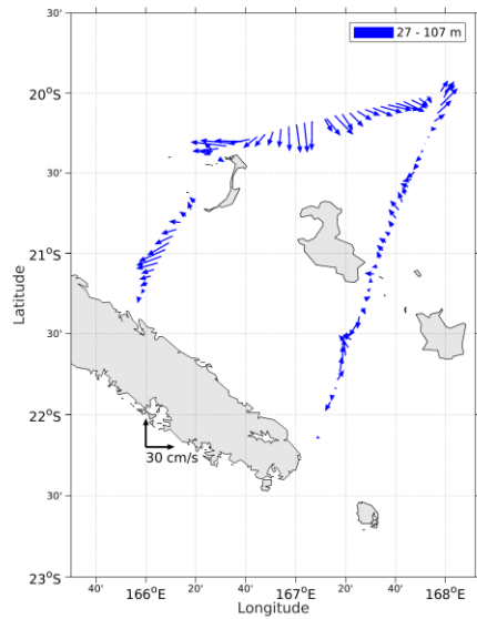
Figure 27- Vecteurs du courant de 0 à 100m
