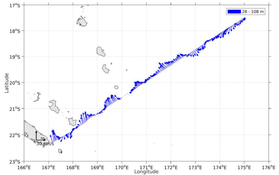
Figure 6- Vecteurs du courant de 0 à 100m
