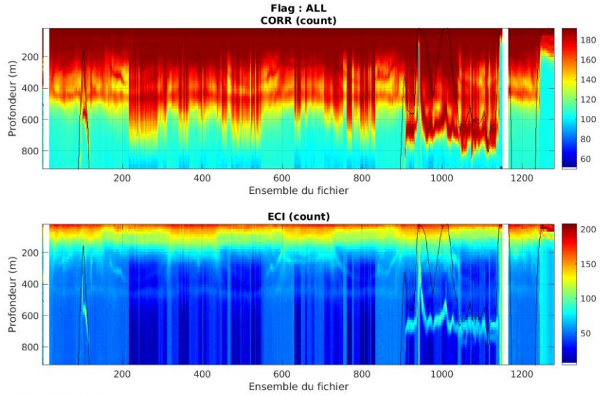
Figure 24 – Indicateur de corrélation (graphe haut) et intensité de l'écho rétro-diffusé (graphe bas) pour tous les flags qualité
