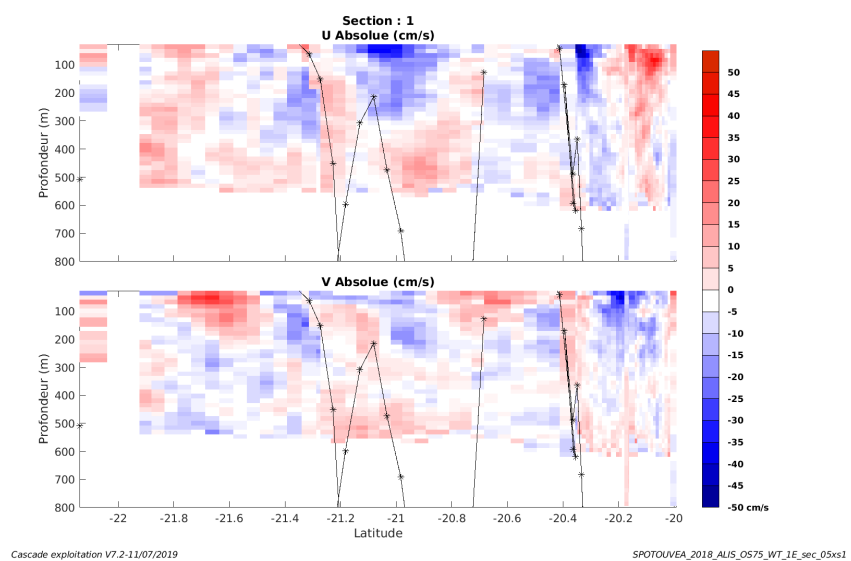
Figure 26 – Composantes du courant – Section 1 de la campagne de 0 à 800 m
