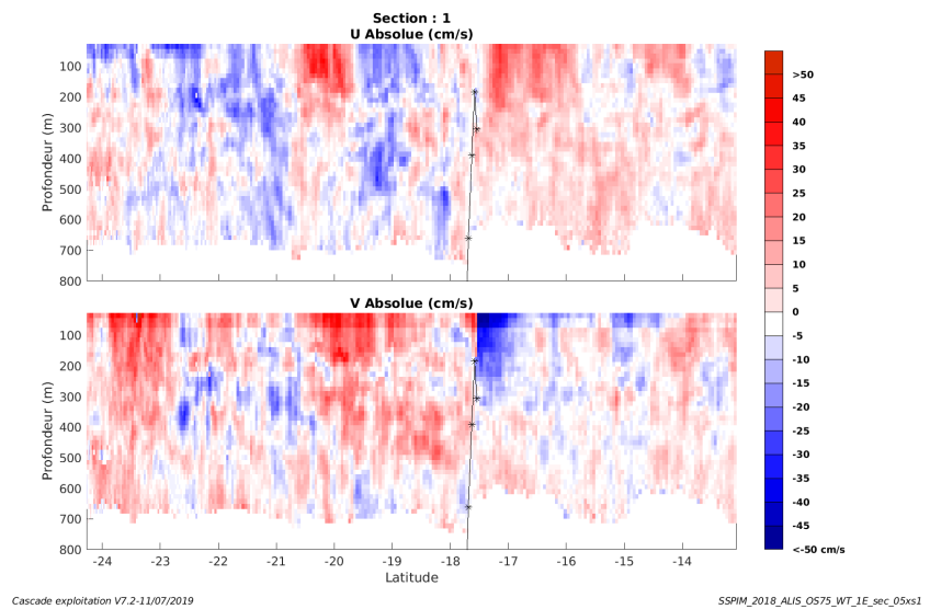
Figure 19 – Composantes du courant – Section 1 de la campagne de 0 à 800 m
