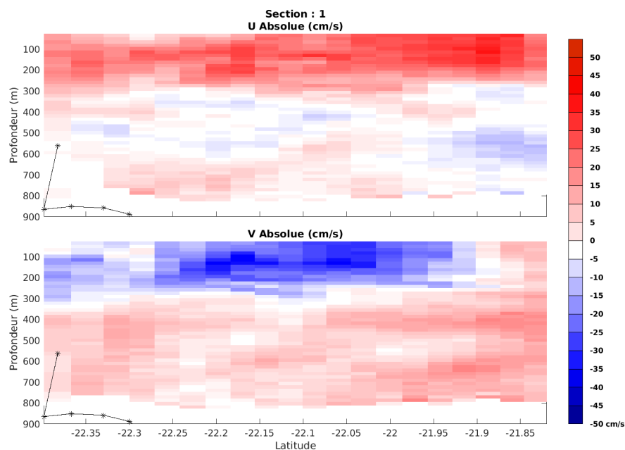
Figure 4 – Composantes du courant – Section 1 de la campagne de 0 à 900m
