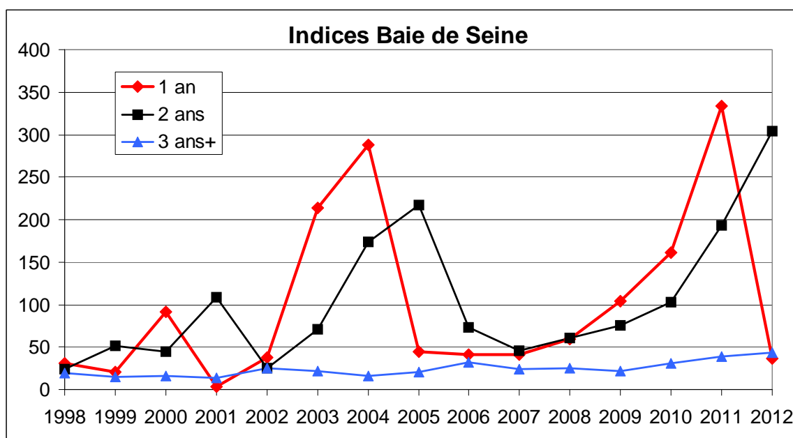
Figure 9 : Biomasse exploitable pour le gisement classé de la baie de Seine et pour l'extérieur de la baie de Seine de 1998 à 2012, et captures estimées (en tonnes) pour la baie de Seine (les valeurs de 1998 à 2011 sont calculées en comparant la biomasse exploitable une année N et le reliquat restant l'année N+1, la valeur pour 2012 se base sur la biomasse disponible en 2012 et un indice de reliquat théorique de 33% à l'issue de la saison de pêche 2012-2013).
