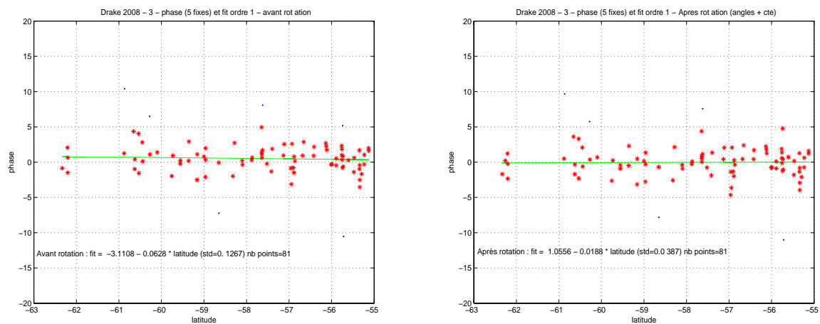
FIG. 6.4 - : DRAKE 2008-3 : Tracé de la phase en fonction de la latitude, avant et après calibration
