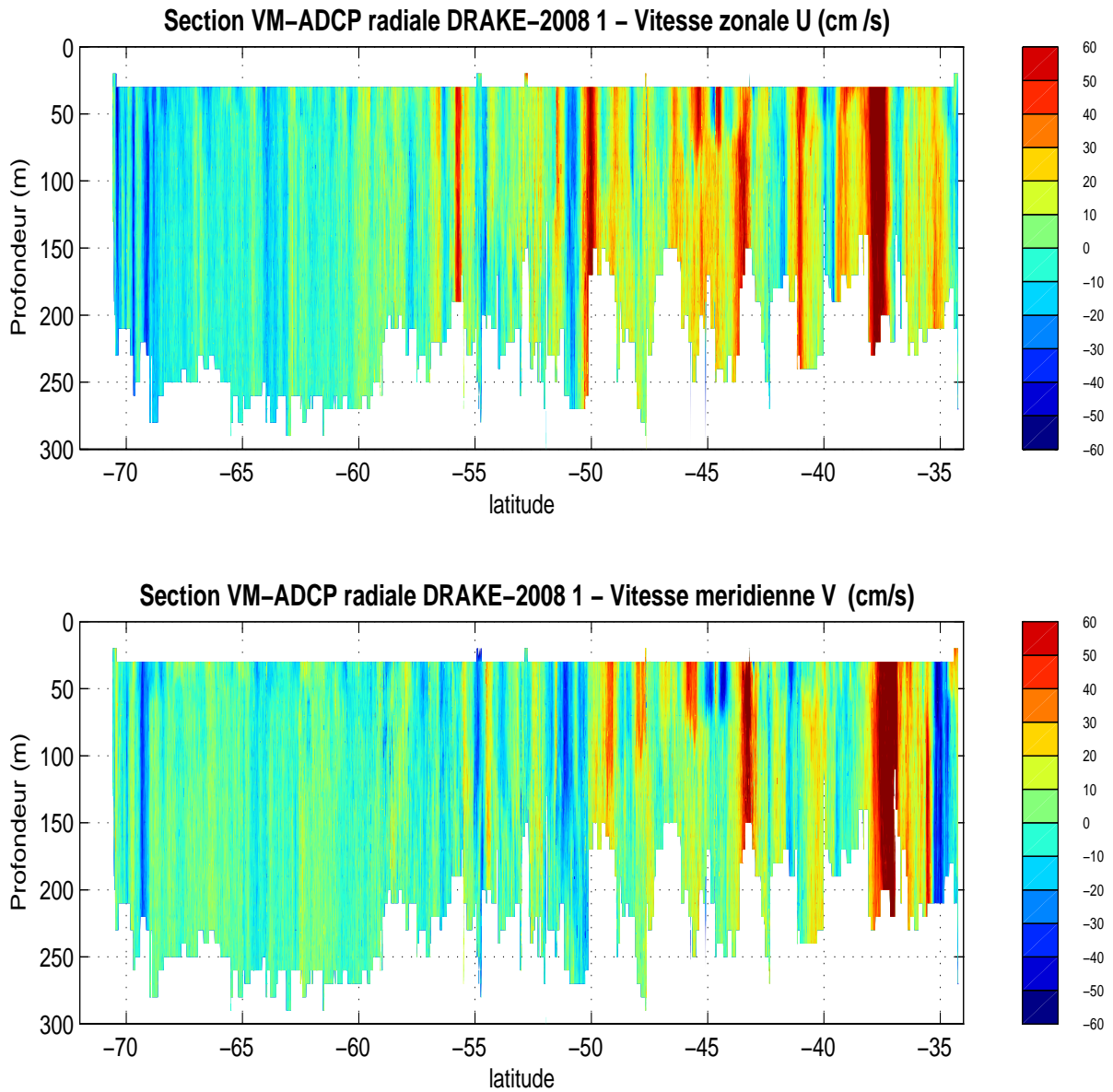
FIG. 7.2 —: Section en latitude pour la radiale aller DRAKE 1
