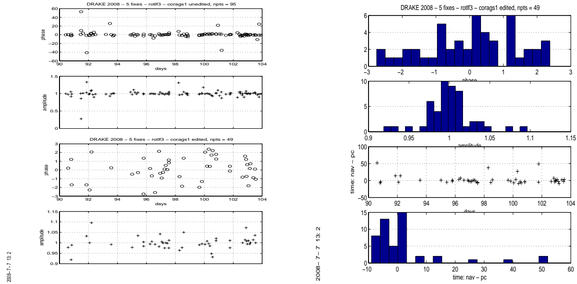
FIG. 6.5 – Détermination de la phase, de l'amplitude et d'un décalage d'horloge
