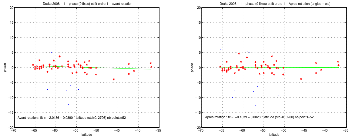
FIG. 6.2 - : DRAKE 2008-1 : Tracé de la phase en fonction de la latitude, avant et après calibration
