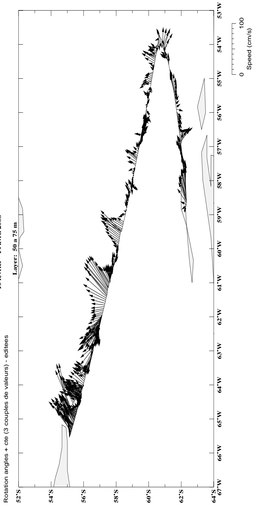
FIG. 7.5 — Vecteurs de courant dans la couche 20 - 50 m pour la radiale DRAKE-2008 3
