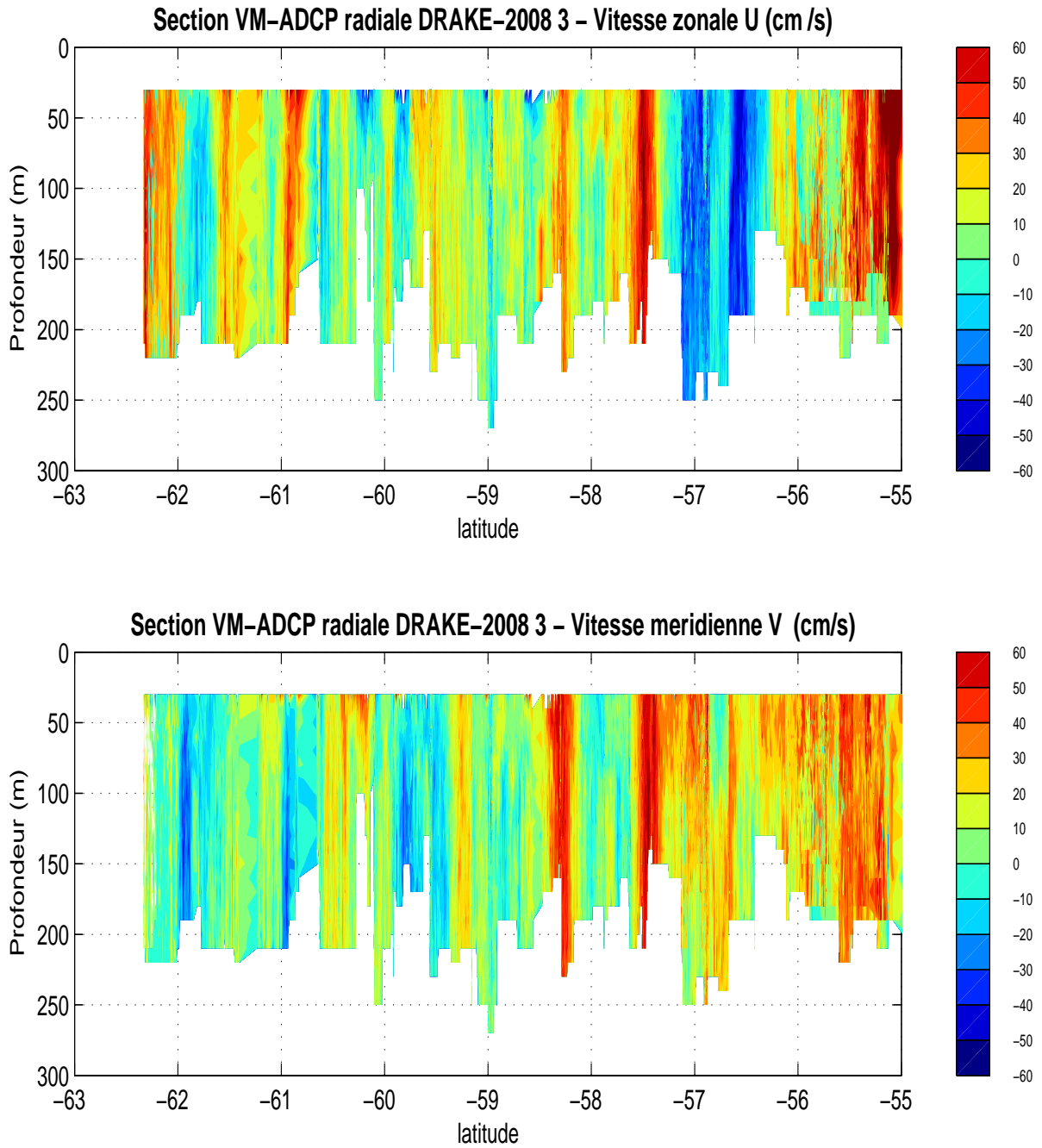
FIG. 7.6 —: Section en latitude pour la radiale DRAKE-2008 3
