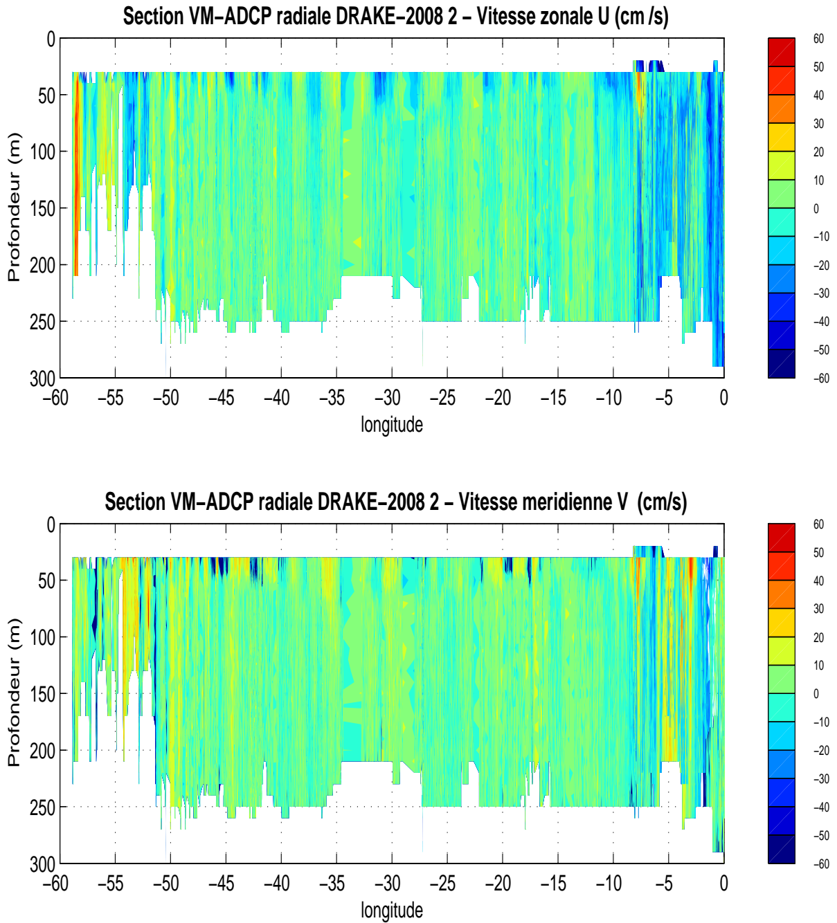
FIG. 7.4 – Section en longitude pour la radiale DRAKE-2008 2
