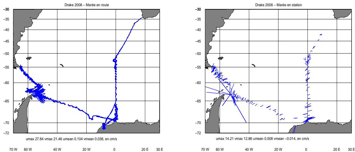
FIG. 6.7 —: Tests de l'influence de la marée en route (à gauche) et en station(à droite)
