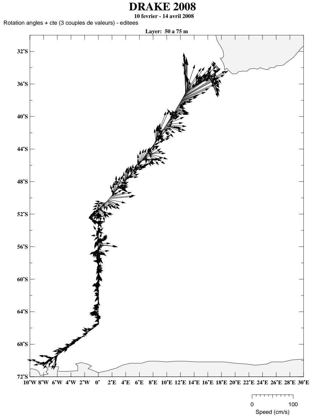
FIG. 7.1 — Vecteurs de courant dans la couche 20 - 50 m pour la radiale DRAKE-2008 1
