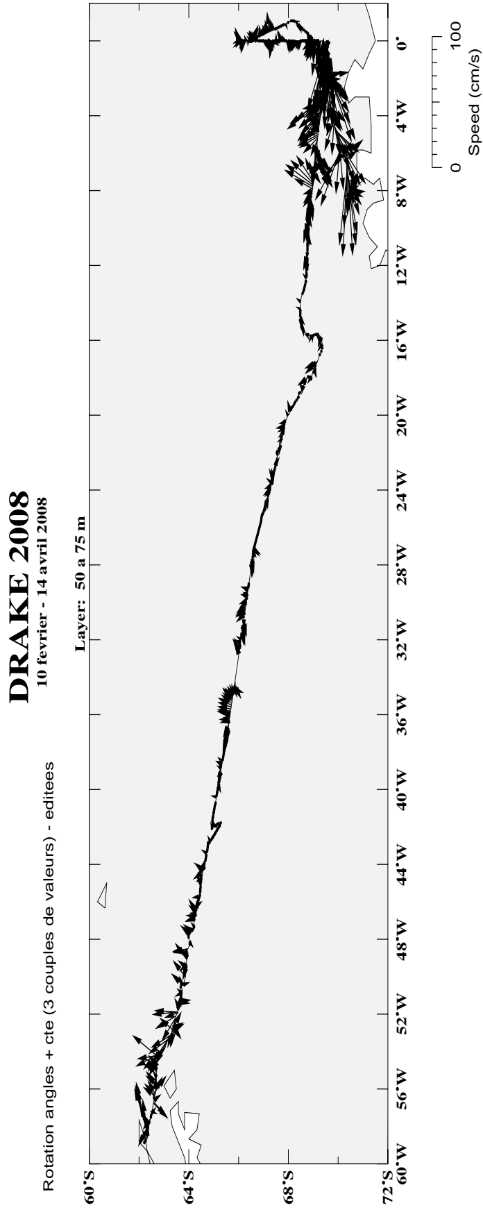
FIG. 7.3 — Vecteurs de courant dans la couche 20 - 50 m pour la radiale DRAKE-2008 2
