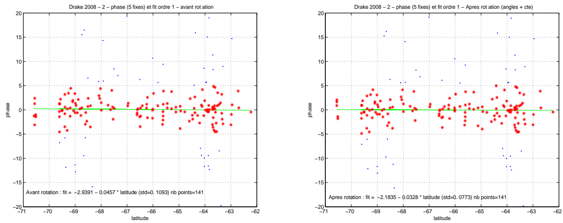
FIG. 6.3 - : DRAKE 2008-2 : Tracé de la phase en fonction de la latitude, avant et après calibration
